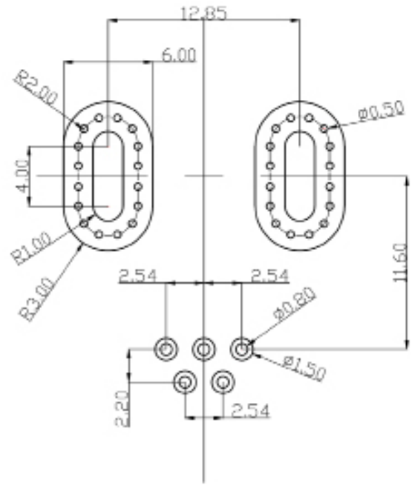
C03-50AH/C03-50AH40
